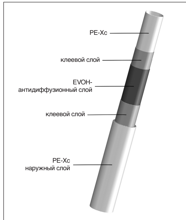
„Сорех“ PE-Xc Полиэтиленовые трубы (диаметры 14 x 2 мм, 16 x 2 мм, 17 x 2 мм, 20 x 2 мм)
