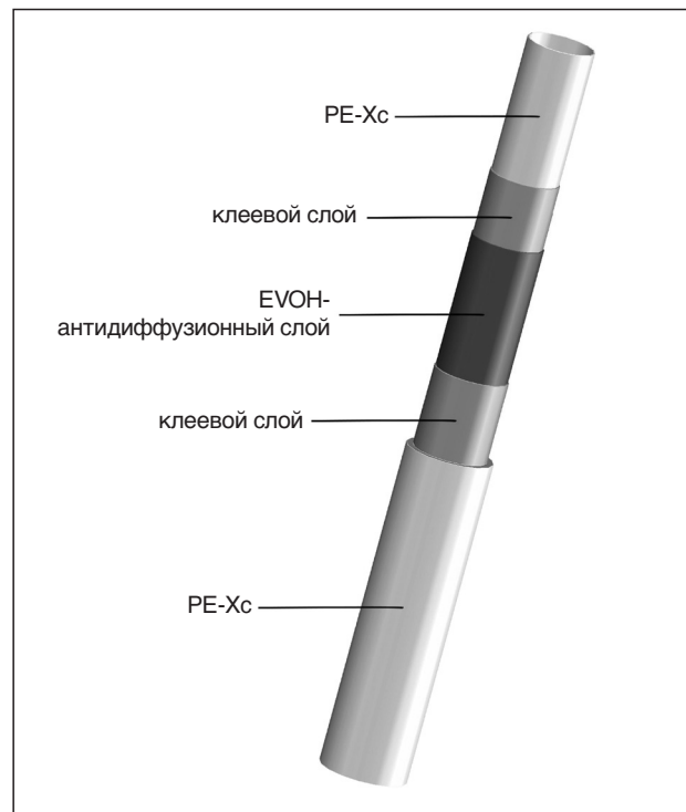
„Сорех“ PE-Xc Полиэтиленовые трубы (диаметры 20 x 2,5 мм, 26 x 3 мм, 32 x 3 мм)
